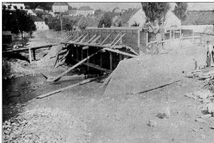
Mostek v roce 1905 během výstavby
