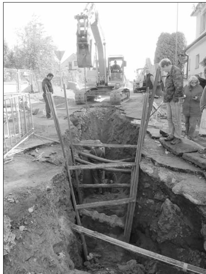
Křížení sítí při výstavbě kanalizace v Nové ulici (foto Martin Hujer)
